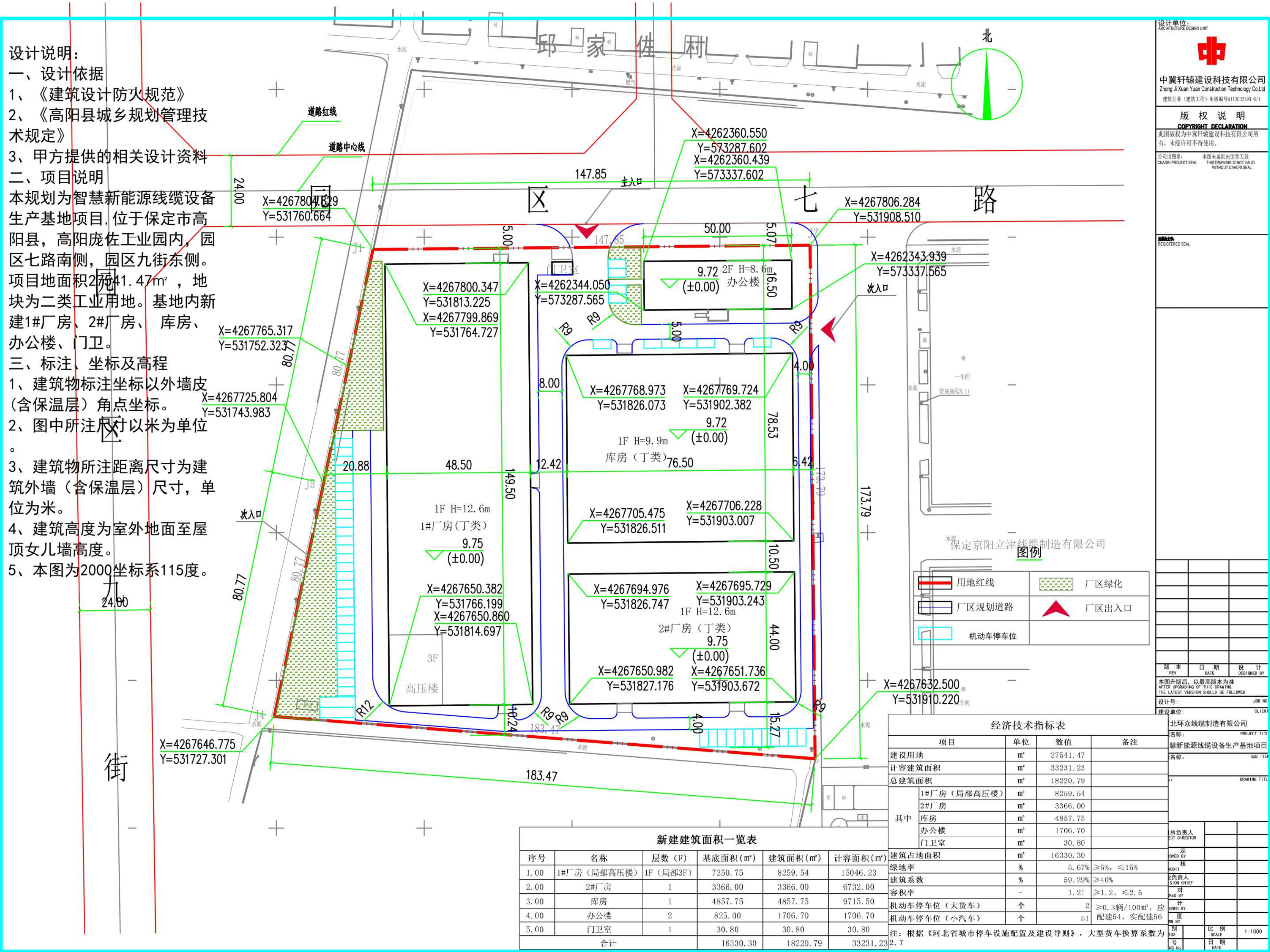
俯视图
